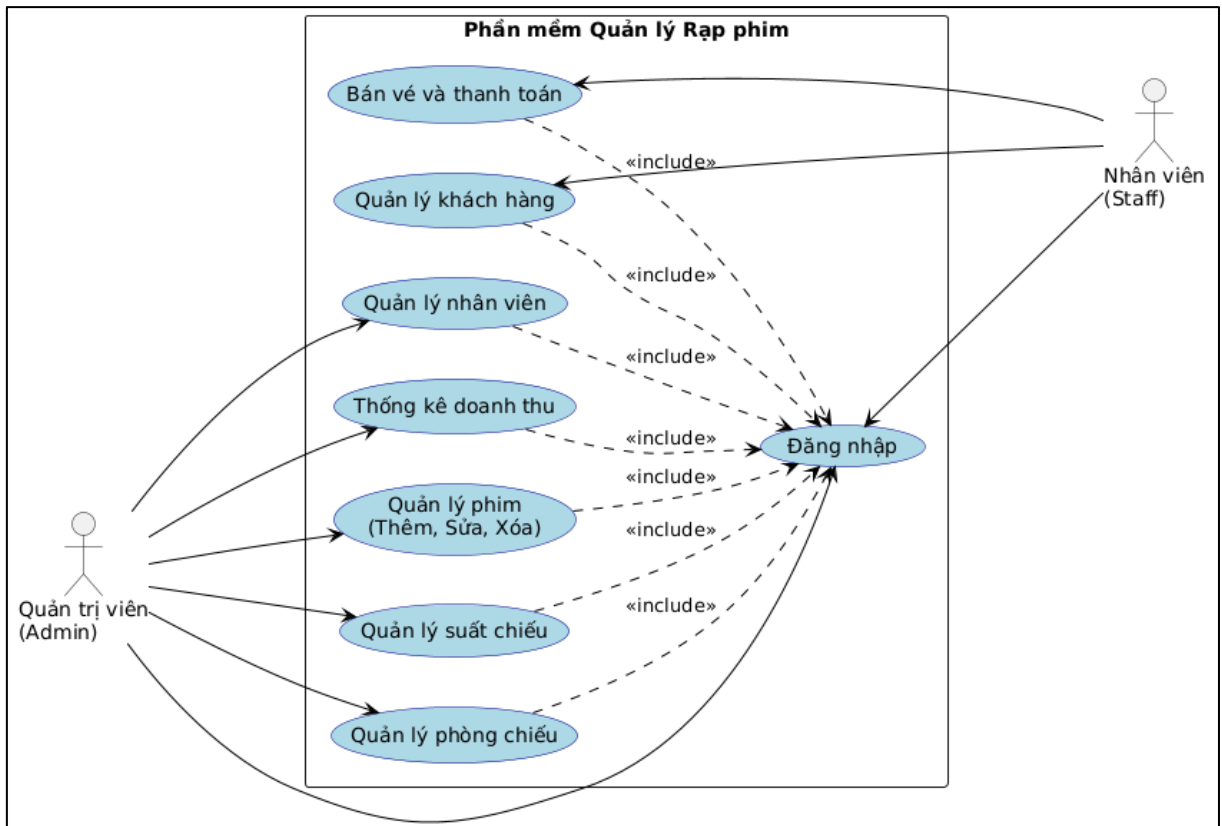
Hình 2.1. Sơ đồ ca sử dụng tổng quát
