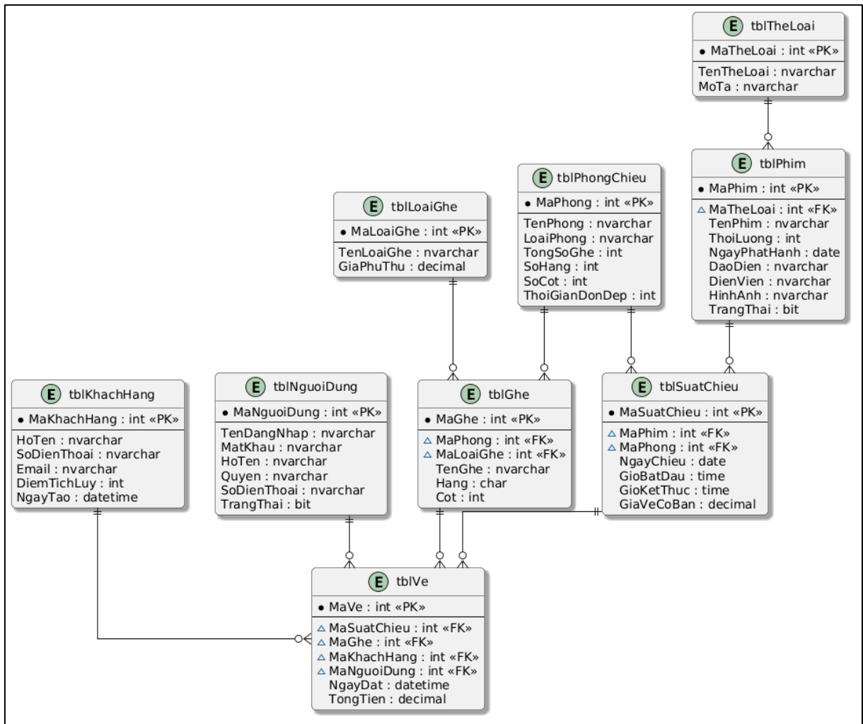
Hình 2.3. Mô hình liên kết
