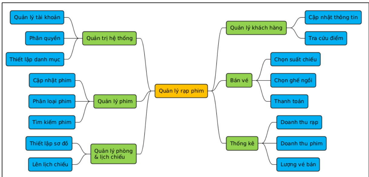
Hình 2.2. Sơ đồ phân cấp chức năng của hệ thống
